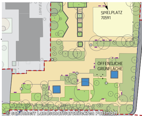
Bestandsplan Brunnenplatz
